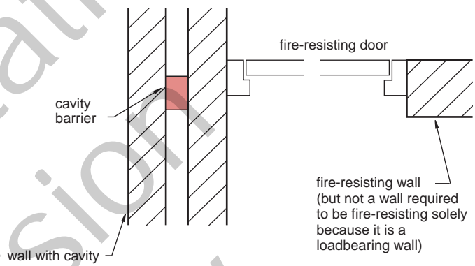
(d) Plan
